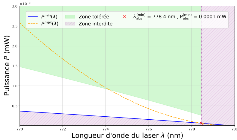
FIGURE VII.6 – Puissance requise en fonction de la longueur d’onde pour w_0 = 1 \mu m
