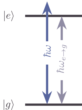
FIGURE VII .1 – Structure à deux niveaux : |g\rangle pour l'état fondamental ("ground") et |e\rangle pour l'état excité ("excited"). La différence d'énergie entre les deux niveaux, notée \hbar\omega_{e\rightarrow g} , est représentée, ainsi que la transition induite par le couplage laser de fréquence \omega . Dans cet exemple, la transition est dans le bleu.
